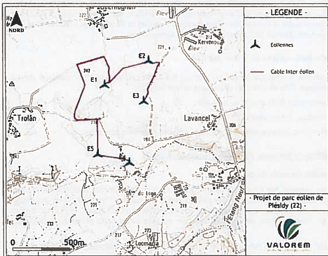
Cheminement pressenti pour le raccordement électrique inter-éolien (source : étude d'impact)
